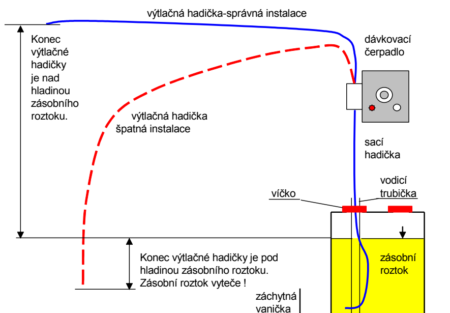
Obrázek č. 1: Příklad správné a špatné instalace dávkovacího čerpadla
